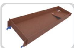
Plateforme de travail avec structure en aluminium, plinthes de 25cm et trappe de passage.
