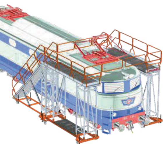
EM207 Structure sur mesure
