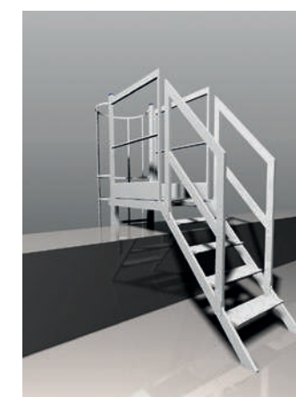
SCALA DISCESA FRONTALE PER PIATTAFORMA DI SBARCO (DISCESA ALL'AVANTI) (aggiungere al prezzo della piattaforma con parapetto cod. 20965 il prezzo della scala a giorno cod 20967). Rampe avec plateforme pour l'accès et la sortie de l'échelle.
